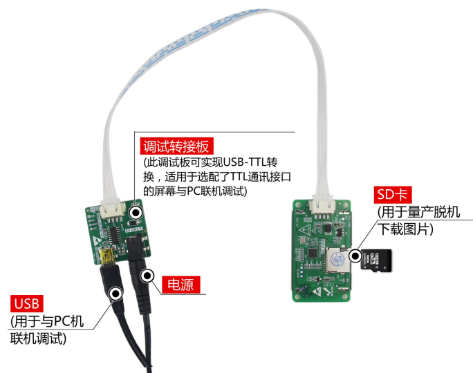
图 1-3 调试工具图
